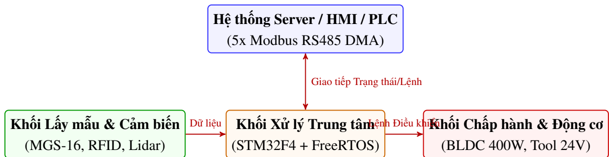
Hình 3.1 Cấu trúc tổng quan của hệ thống xe tự hành AGV B400.
